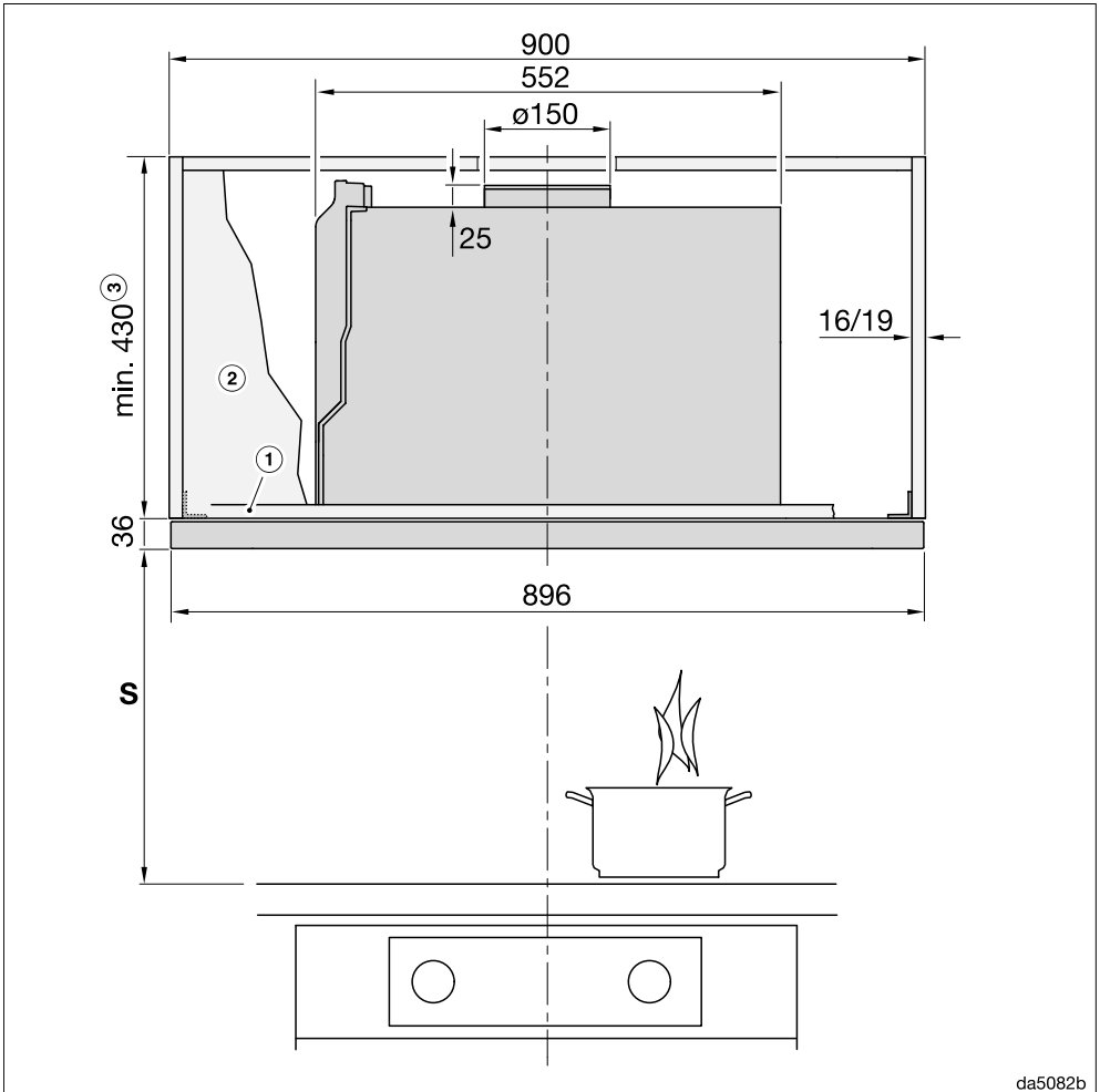
2. attēls: DAS 4930 ir ievietots 900 mm platā skapī
