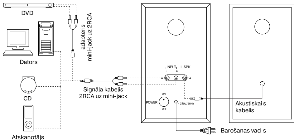
Zīmējums 2. Pieslēgšanas shēma.
